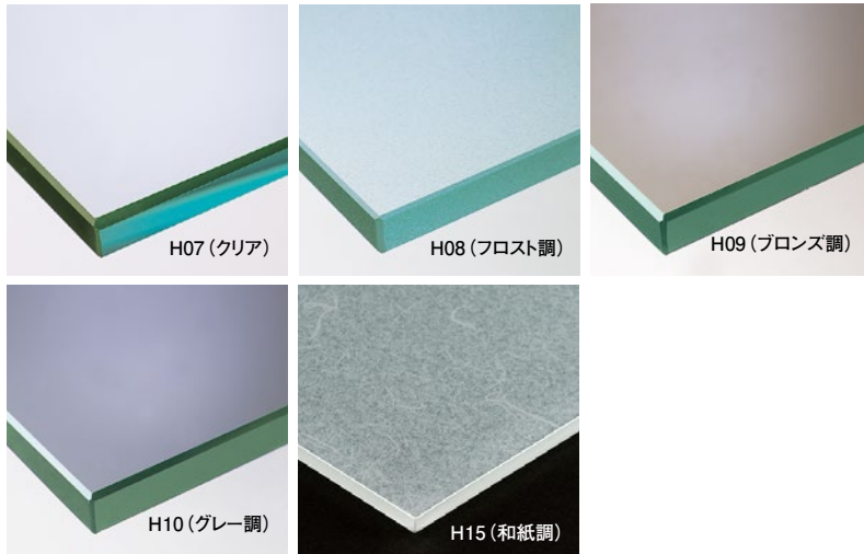
飛散防止フィルム貼り (H08) ガラス天板 W1200×D600/450×8mm厚 テーブル脚 YG-56st
