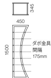
図面はEM(MT)-26/27・MA-26/27共通です。
