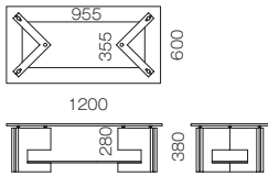
MS(MSW)-2 ● W1200×D600×H380mm／総重量34.2kg ● フレーム:天然石 (マクタンストーン)、ステンレス ● 天板:透明ガラス10mm／棚板:透明ガラス8mm 天板～棚板まで280mm ¥100,000 (本体価格) ※2023年9月価格改定
