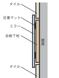
断面図 ①
