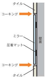
断面図 ②
