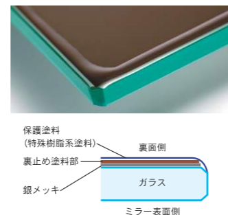
糸面取り小口磨き 最もベーシックな小口処理です。 巾広面取り小口磨き 15mm幅が標準です。
