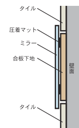
断面図 ①
