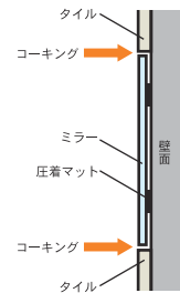
断面図 ②
